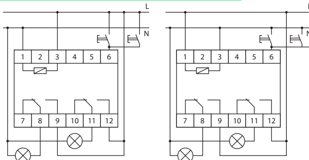
Кнопки управления подключены к фазному проводу L.
