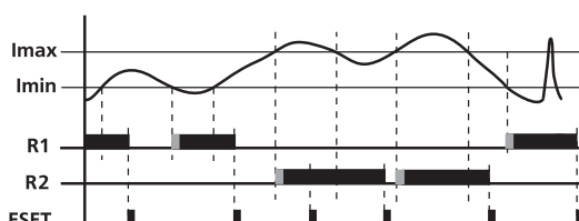
Функция D: если ток меньше I_{min} , замкнуты контакты R1. При достижении значения тока I_{max} замыкаются контакты R2. Контакты реле блокируются до момента нажатия кнопки RESET на лицевой панели.
