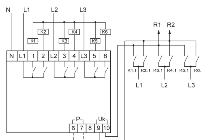
С применением контакторов.
