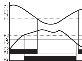
Программа 5. Охлаждение
