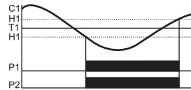
Программа 1. Нагрев
