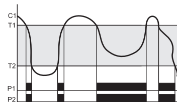
Программа 8. Работа в режиме «Окно»
