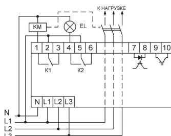
Схема включения ОМ-630, ОМ-630-1.
