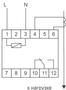
Схема подключения
