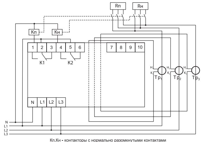
Кп, Кн - контакторы с нормально разомкнутыми контактами
