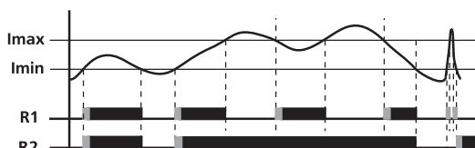
Функция В: если ток больше I_{min} , замкнуты контакты реле R1 и R2, при токе больше I_{max} контакты R1 размыкаются.
