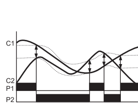
Программа 7. Работа в зависимости от разности температур C1 и C2
