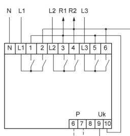
Без применения контакторов.
