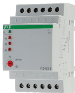
Трёхуровневый с регулировкой чувствительности.
