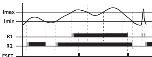
Функция С: если ток больше I_{min} , замкнуты контакты реле R2, если ток больше I_{max} , замкнуты контакты реле R1. Реле R1 блокируется до момента нажатия кнопки RESET на лицевой панели.
