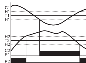
Программа 4. Нагрев
