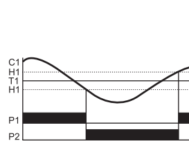
Программа 3. Нагрев/Охлаждение
