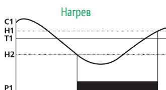
Диаграммы работы CRT-05
