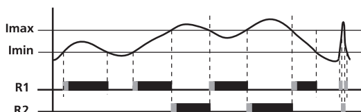
Функция А: если ток больше I_{min} , замкнуты контакты реле R1, при токе больше I_{max} замкнуты контакты реле R2.
